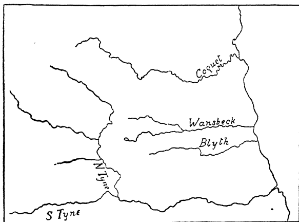
चित्र १७२—नार्थम्बरलैण्ड की नदियाँ।
